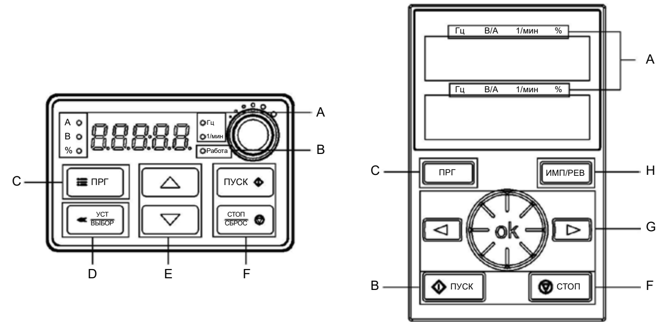
Рисунок 4.1-1 Панель управления преобразователя частоты и выносная цифровая панель
