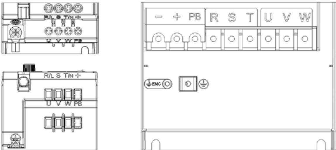
Рисунок 3.1-2 Расположение клемм
